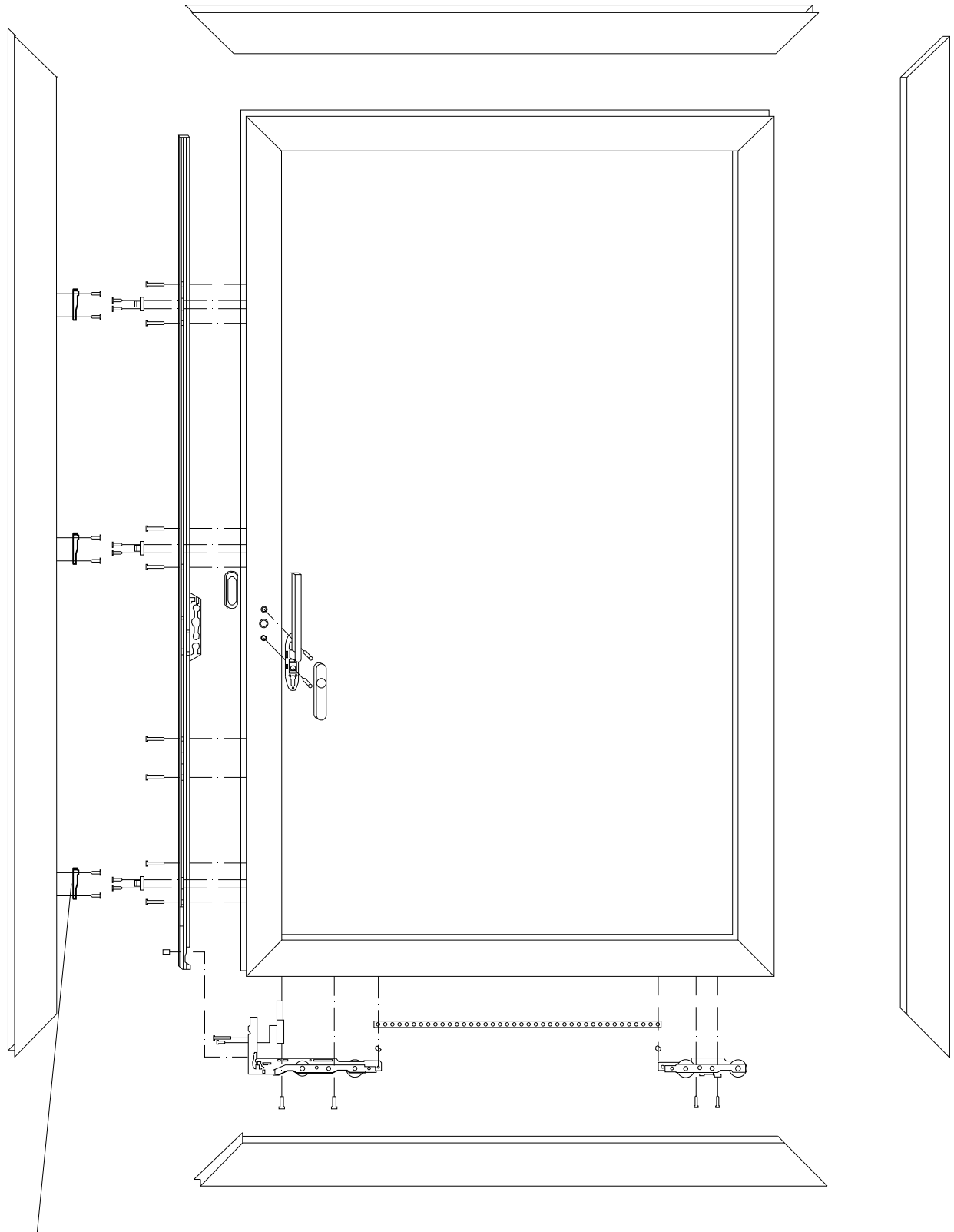
CERRADERO UNIVERSAL
