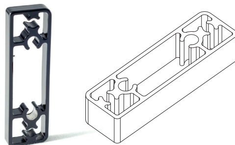
PROIN148 Calzo para bisagra solo para aplicaciones en aluminio
