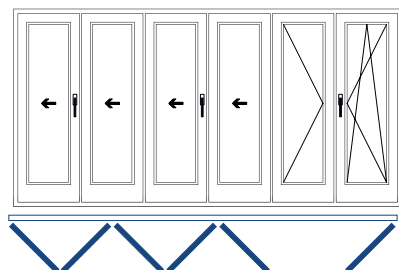
651 5 bastidores plegables 1 bastidor de paso [1]
