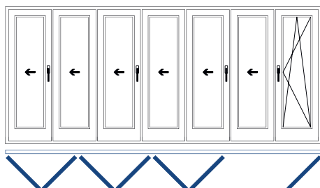
761 6 bastidores plegables 1 bastidor de paso [1]
