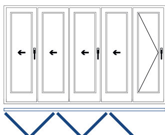
550 4 bastidores plegables 1 bastidor de paso
