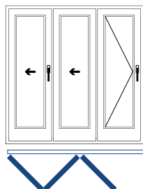
330 2 bastidores plegables 1 bastidor de paso
