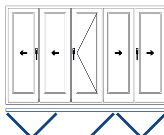
532 2 bastidores plegables/1 de paso 2 bastidores plegables
