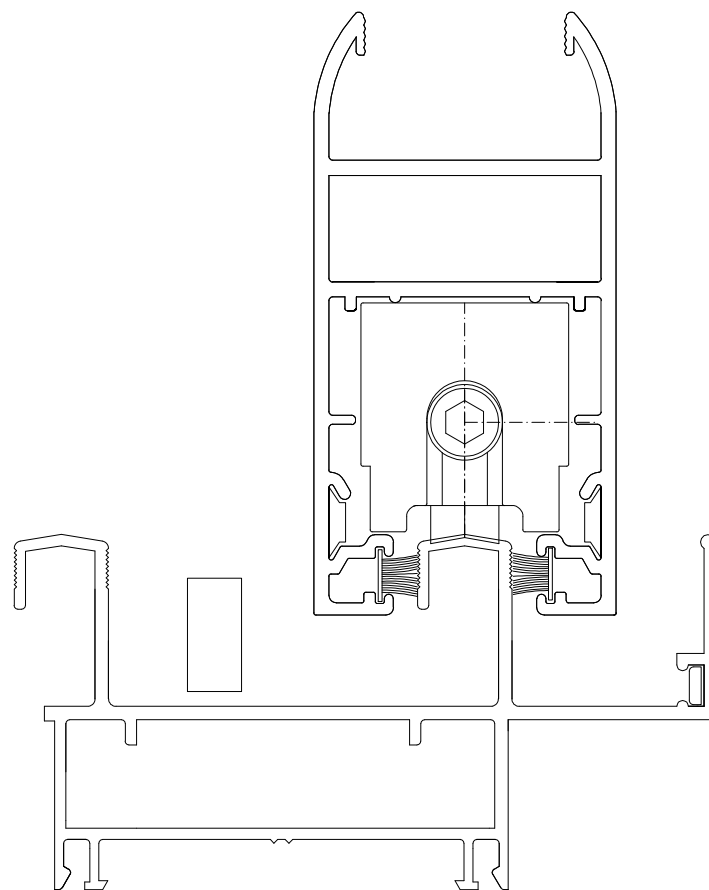
Instalação - escala 1:1
