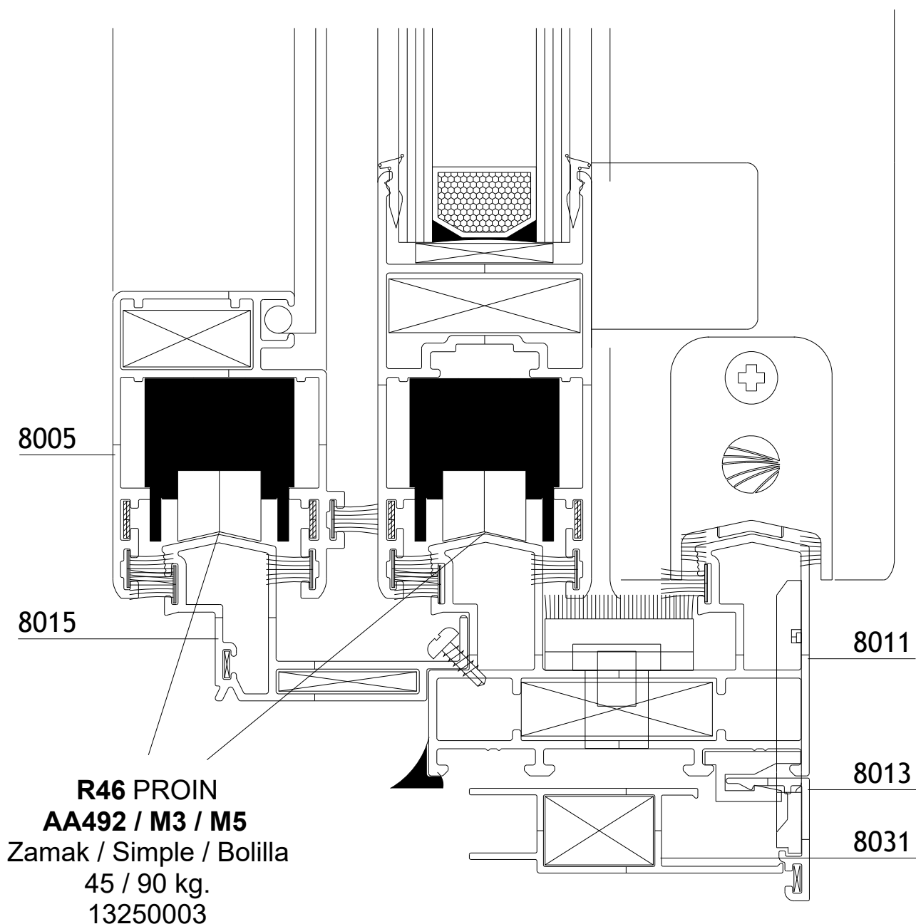
CORTE 4-5
