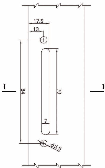
DETALLE A CALADO DE PERFIL PARA FALLEBA
