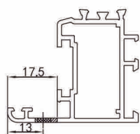
CORTE 1-1
