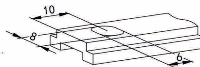
PUNZONADO PLETINA
